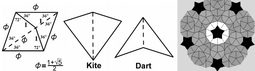
Плитки мозаики Пенроуза.
