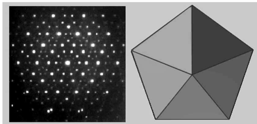
Электронограмма непериодического кристалла с осью симметрии пятого порядка.
