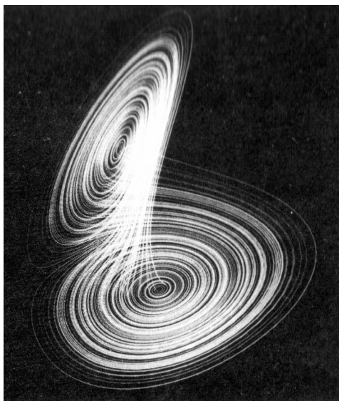
Странный аттрактор Лоренца.
